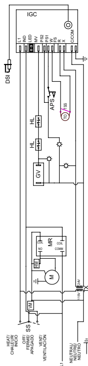
ELECTRICAL LADDER DIAGRAM / DIAGRAMME EN ESCALIER / DIAGRAMA ELECTRICO DE ESCALERA
