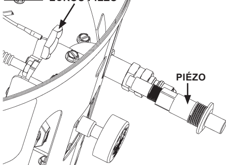
FIG. 18 ÉCROU PIÉZO
