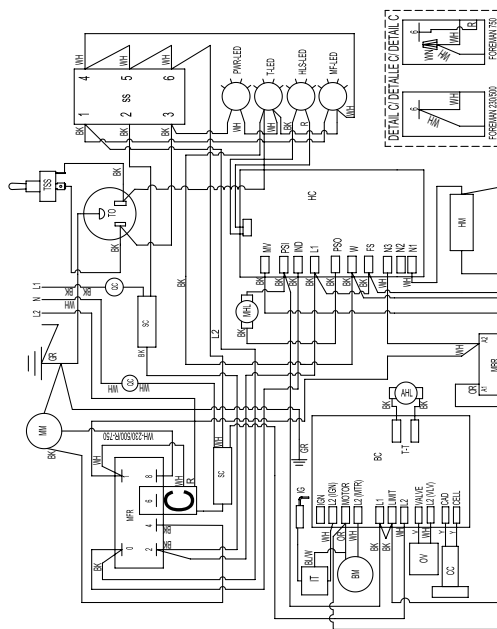
ELECTRICAL CONNECTION DIAGRAM / CONNEXIONS ELECTRIQUES / DIAGRAMA DE CONEXIONES ELECTRICAS
