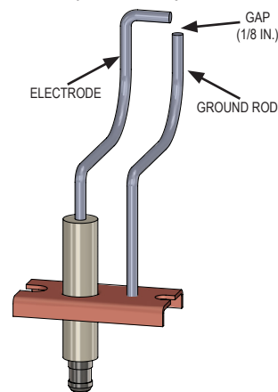
FIG. 16 (ST60/ST80)
