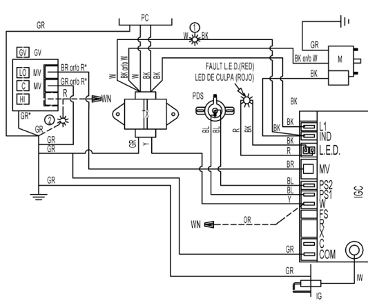
ELECTRICAL CONNECTION DIAGRAM / DIAGRAMA DE CONEXIONES ELÉCTRICAS
