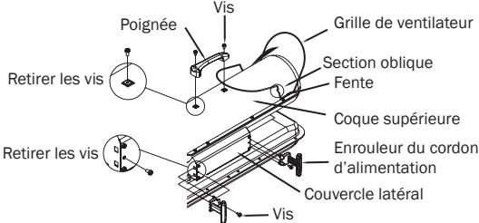
Figure 4 - Installation de la poignée et de l'enrouleur du cordon d'alimentation
