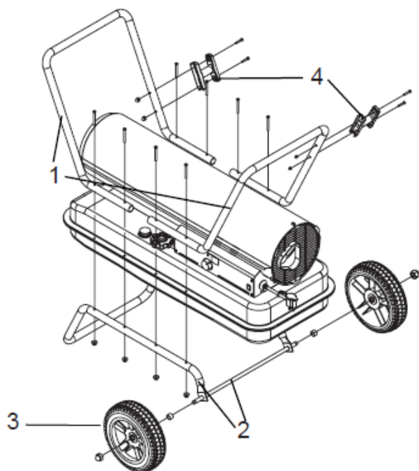
Figure 30– Illustration des pièces de rechange pour les modèles CP125FK, CP175FK, CP220AK
