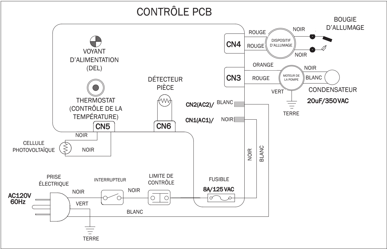
Figure 26 – Diagramme de câblage modèles CP125FK, CP175FK, CP220AK
