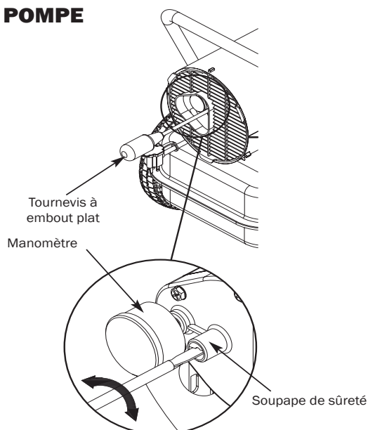
Figure 22 – Ajustement de la pression de la pompe
