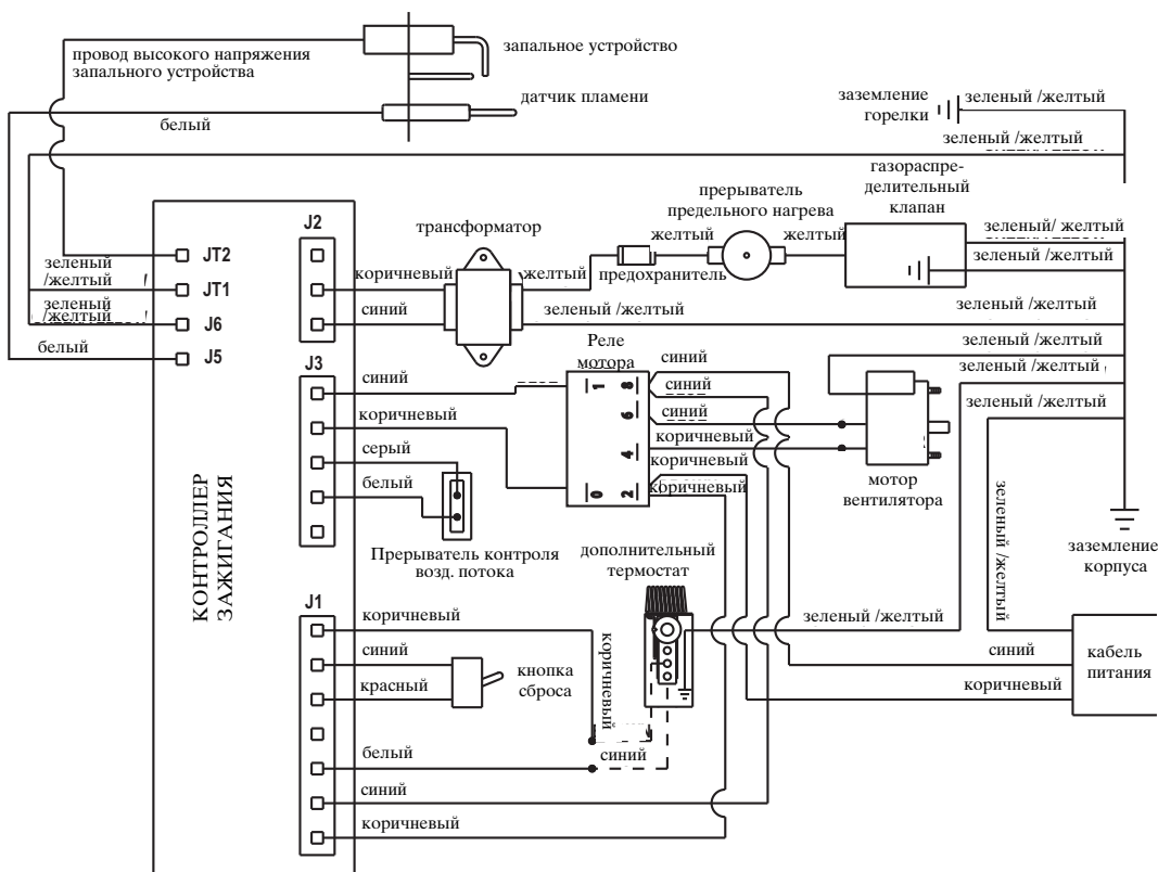
Диаграмма подключений
