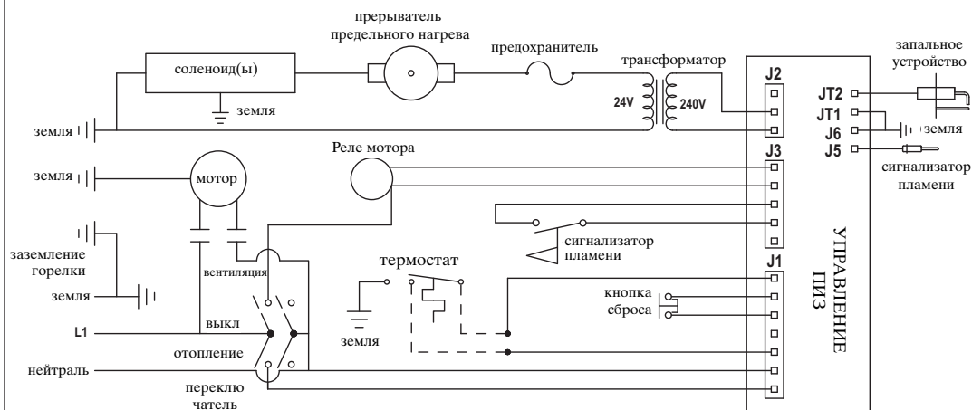
Развернутая схема
