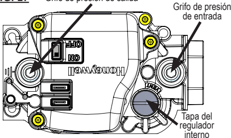
FIG. 27 Grifo de presión de salida
