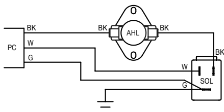
ELECTRICAL CONNECTION DIAGRAM / DIAGRAMA DE CONEXIONES ELÉCTRICAS
