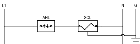
ELECTRICAL LADDER DIAGRAM / DIAGRAMA ELÉCTRICO DE ESCALERA
