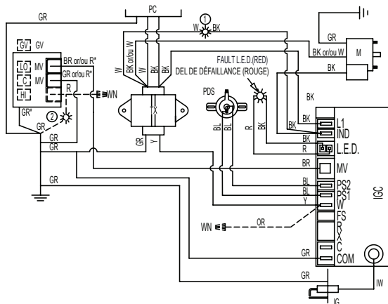
ELECTRICAL CONNECTION DIAGRAM / SCHÉMA DE RACCORDEMENT ÉLECTRIQUE
